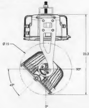
4a Pendant Mount
