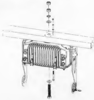
12b Local Pendant Mount
