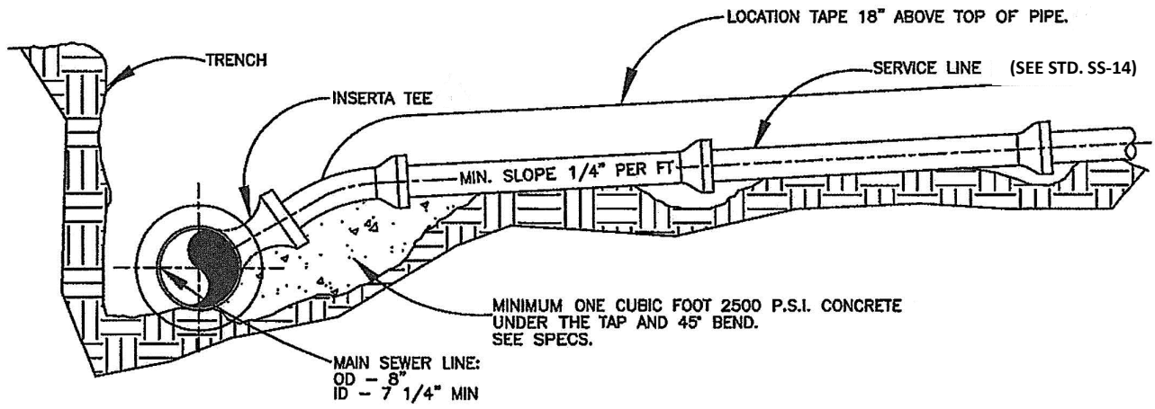
ELEVATION
